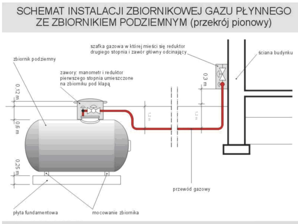
Ryc. 1. Rysunek poglądowy instalacji gazowej zbiornika.
