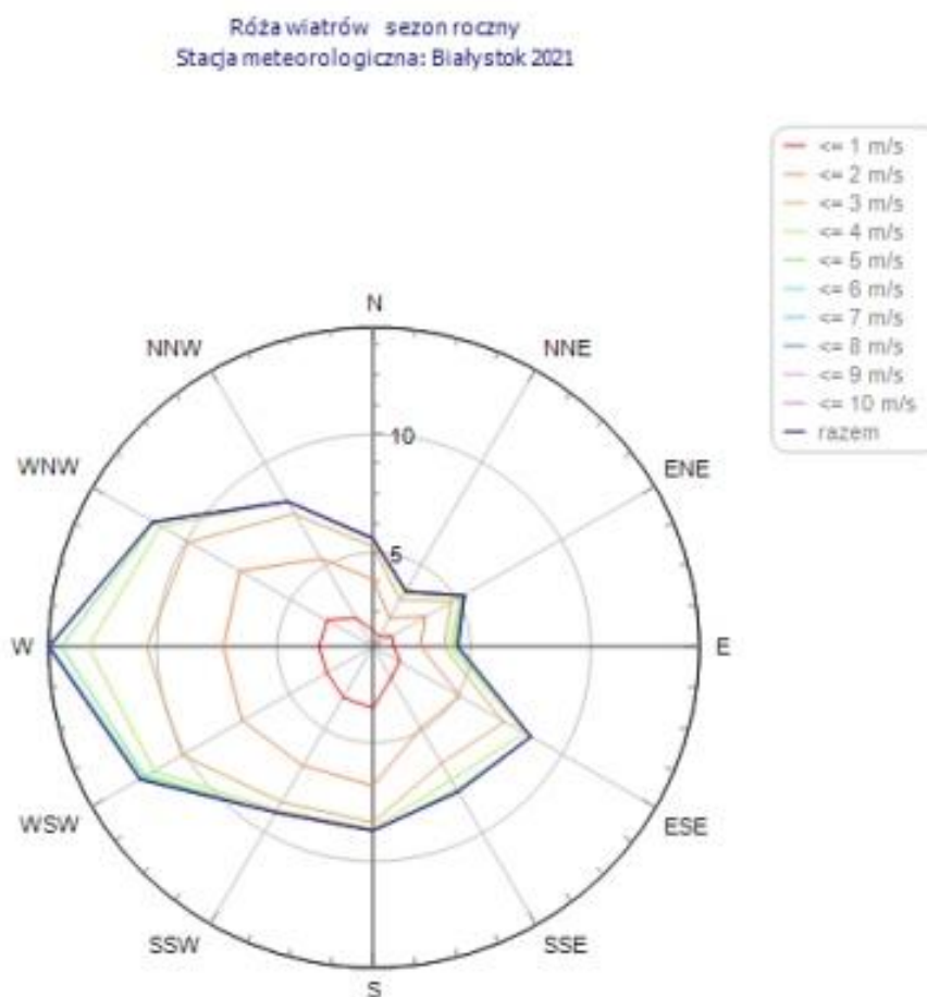
Rys. 2. Róża wiatrów
